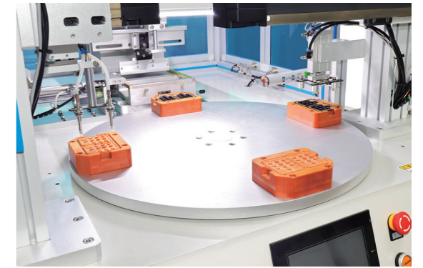
▲ 转盘工作台 Rotary Table Workbench
