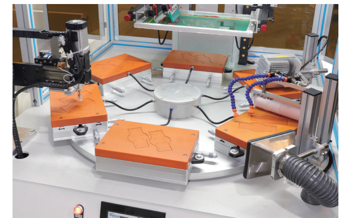
▲ 转盘多工位工作台 Rotary Table Workbench
